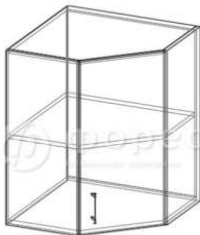
ШВУ-590 (ШxBxГ) 590x716x590 мм
